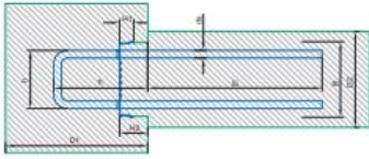
Rückbiegeanschluss zweiarmig
